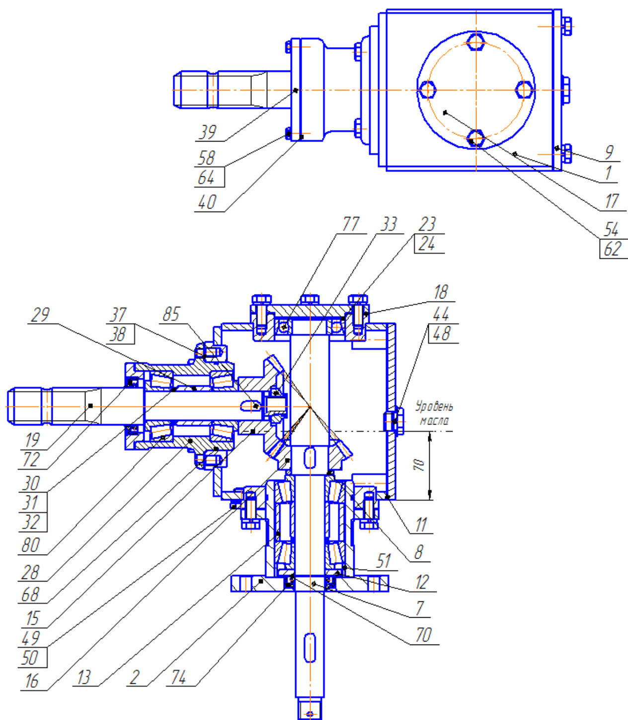
Рис.4 – Редуктор KTC-1.6.11.00.000
