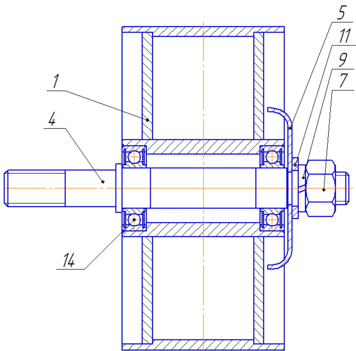
Рис.2 – Колесо КТС-1.6.07.00.000
