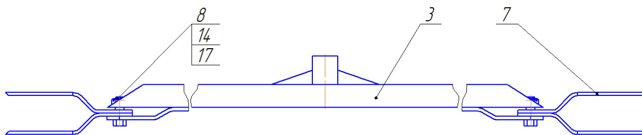
Рис.3 – Нож КТС-1.6.10.00.000
